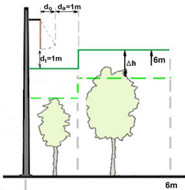
Figura 1. Traversări și apropieri LEA JT față de arbori/pomi fructiferi
