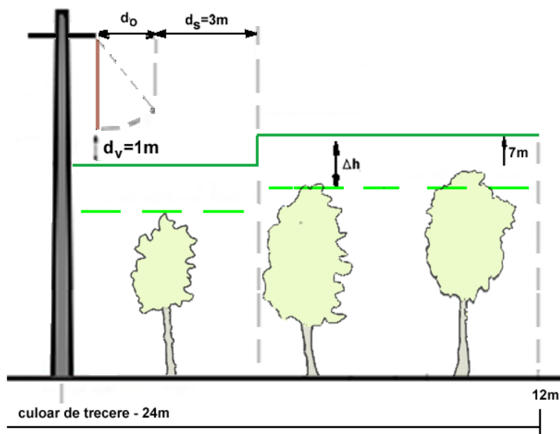
Figura 1.b Profil culoar de trecere LEA 20 kV
