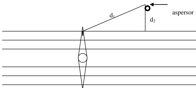
Figura 2. Distanțe minime de amplasare a unui aspersor.
