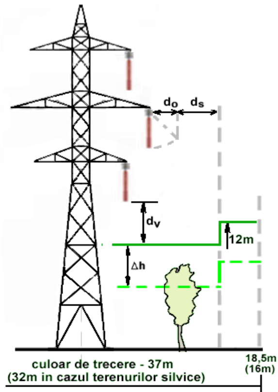
Figura 1.c Profil culoar de trecere LEA 110 kV
