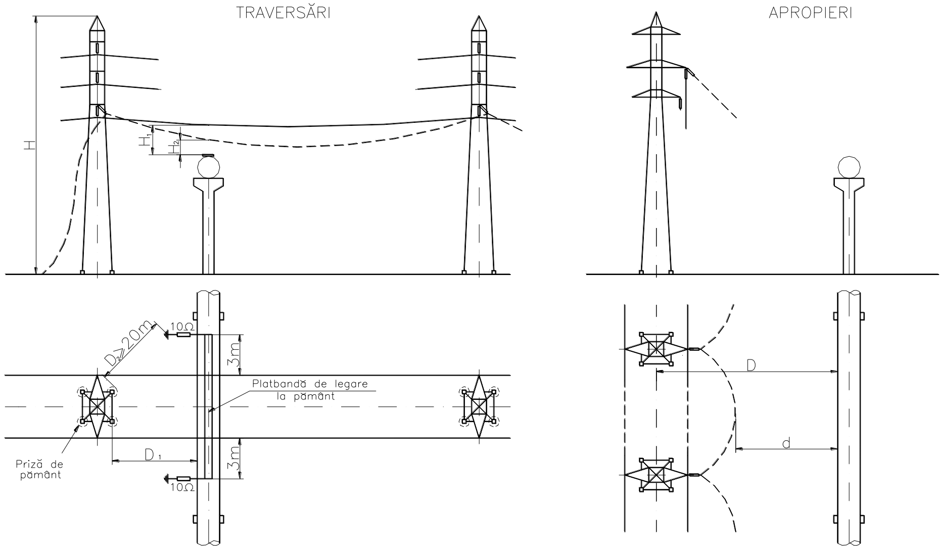
Figura 8. Traversări și apropieri față de conducte supratere
