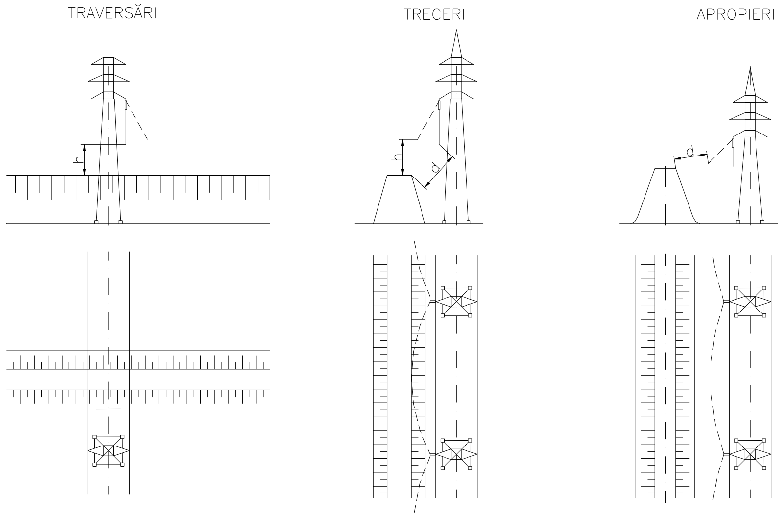
Figura 11.c. Traversări, treceri și apropieri față de diguri.
