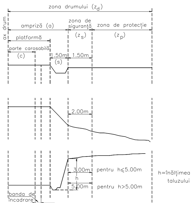
Figura 4. Elemente de gabarit ale drumurilor
