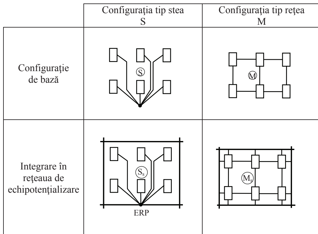
Fig. 4.8. – Integrarea echipamentelor electrice în rețeaua de echipotențializare.
