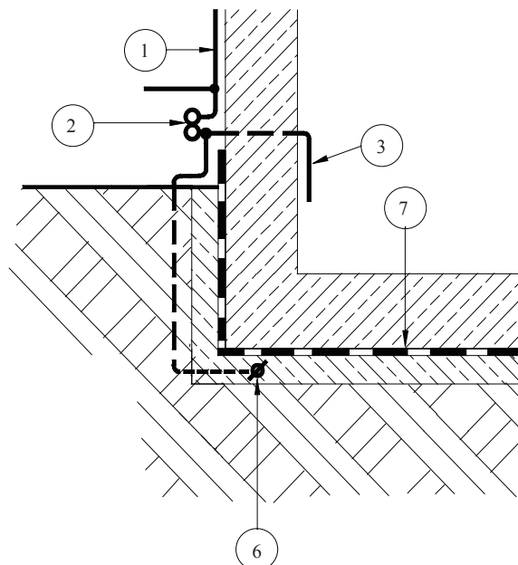
Fig. 6.27 b – Fundație izolată cu conductorul prizei de pământ trecând parțial prin sol
