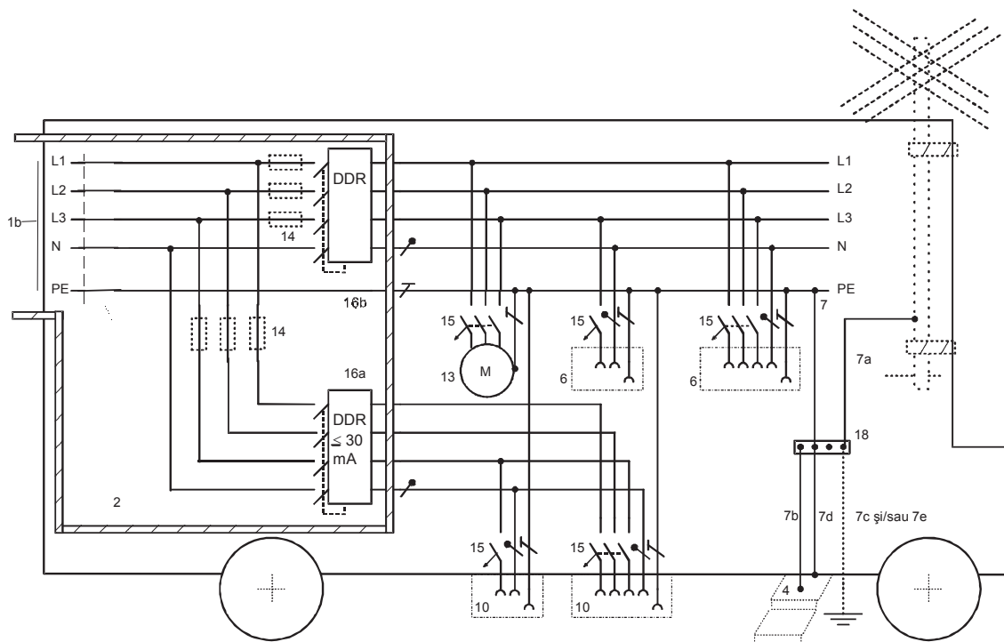
Figura 7.13.3 – Exemplu de conectare la toate tipurile de rețele legate la pământ a unei instalații fixe cu întreruperea automată a alimentării prin dispozitive de curent diferințial rezidual (DDR), cu sau fără priză de pământ
