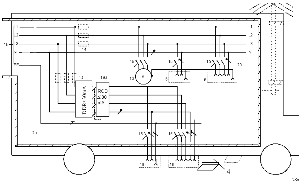
Figura 7.13.4 – Același exemplu cu protecție prin legătură de echipotencializare locală nelegată la pământ cu o carcasă neconductoră în interiorul unității
