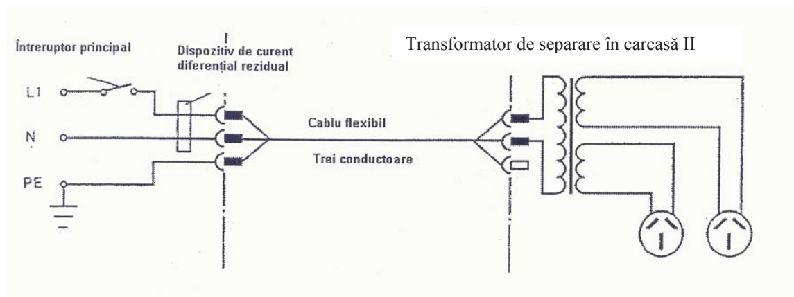
Fig. 7.8.4. Conexiune la rețeaua de alimentare cu dispozitiv de protecție de curent diferențial rezidual prin transformator de separare la bord, fără echipotențializare
