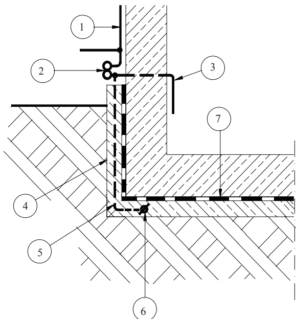
Fig. 6.27 a – Fundație izolată cu electrod de pământ în fundație într-un strat de beton nearmat sub izolația de bitum
