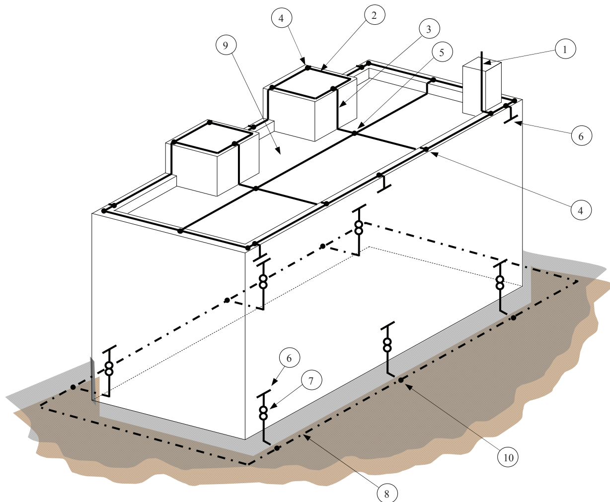
Fig. 6.20 – Construcția unei IPT exterioare pe o structură de beton armat utilizând armăturile pereților exteriori ai structurii drept componente naturale
