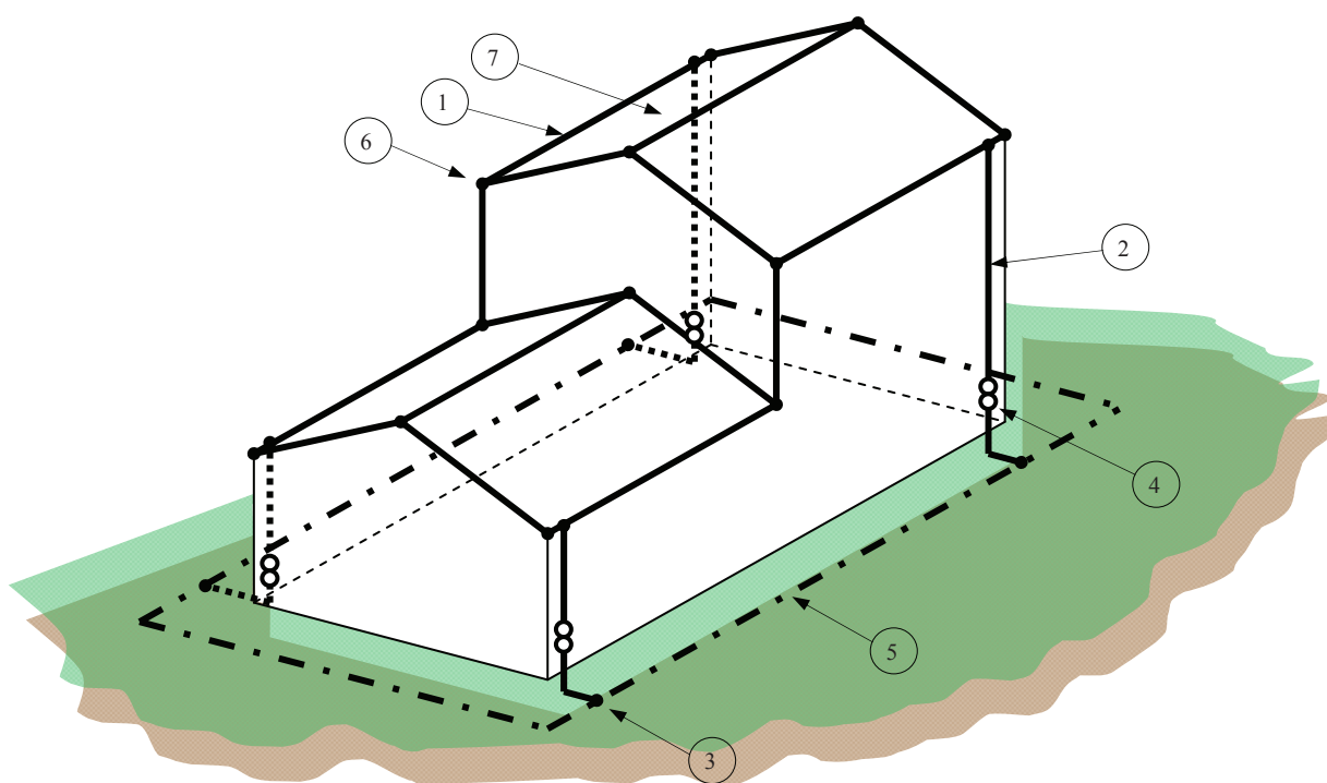
Fig. 6.23 – Construcția unei IPT exterioră pe o structură de material electroizolant cu diferite niveluri de acoperiș
