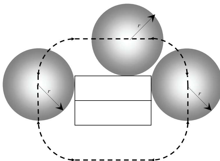
Fig. 6.16 – Puncte de impact ale trăsnetului pe o clădire
